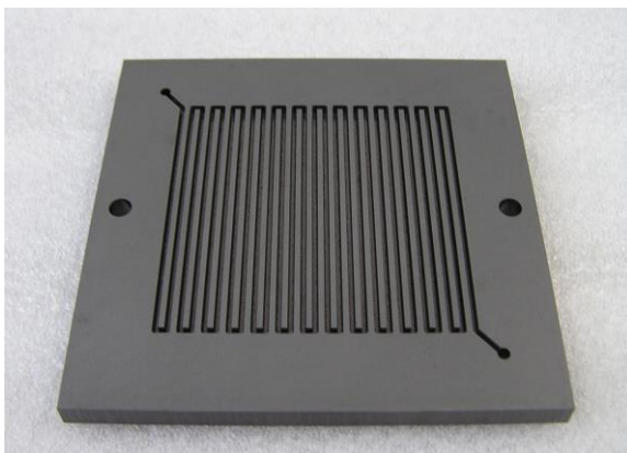
カーボンセパレーター(サーペンタイン) ストレート・オリジナル流路など製作可能
