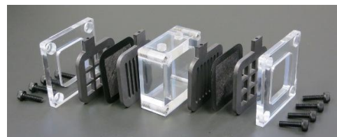
部材構成
