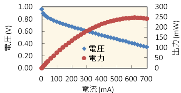
出力特性
