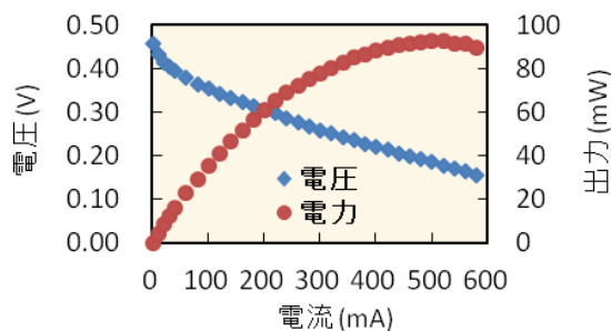
出力特性
